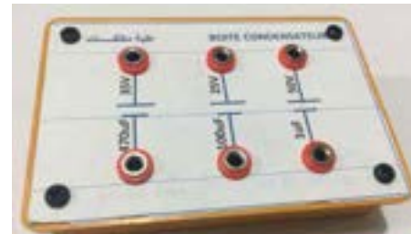
MA-PH 338 BOITE CONDENSATEURS 1100.00 DA
